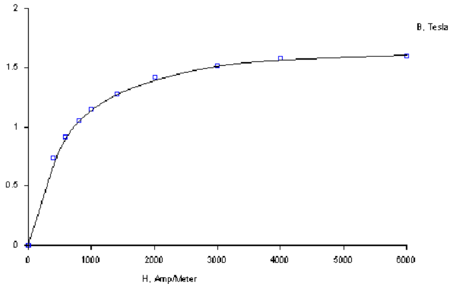
Figura 12 : Curbă de magnetizare trasată de FEMM
